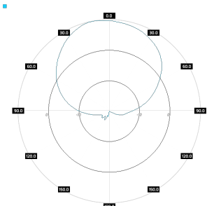
SA M4DBC245-65-9X Slant-pol, elev, 5.5GHz
