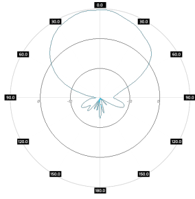
SA M4DBC245-65-9X H-pol, azimuth, 5.5GHz
