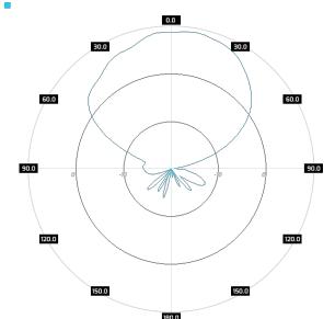
SA M4DBC245-65-9X V-pol, elev, 5.5GHz
