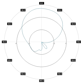
SA M4DBC245-65-9X Slant-pol, azimuth, 2.45GHz
