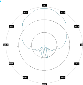
SA M4DBC245-65-9X V-pol, azimuth, 5.5GHz
