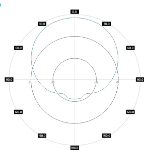
SA M3DBC245-65-9HV H-pol, elev, 2.45GHz
