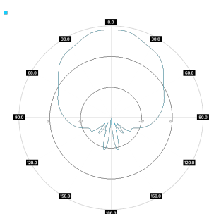
SA M3DBC245-65-9HV V-pol, azimuth, 5.5GHz
