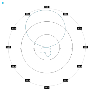
SA M3DBC245-65-9HV V-pol, elev, 2.45GHz
