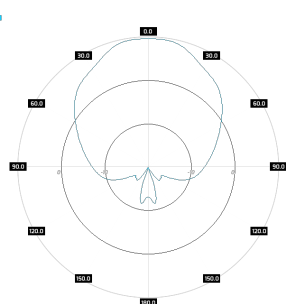
SA M3DBC245-65-9HV H-pol, elev, 5.5GHz
