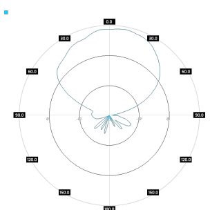
SA M3DBC245-65-9HV V-pol, elev, 5.5GHz
