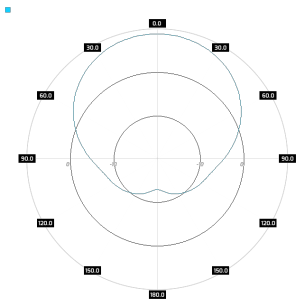
SA M3DBC245-65-9HV V-pol, azimuth, 2.45GHz
